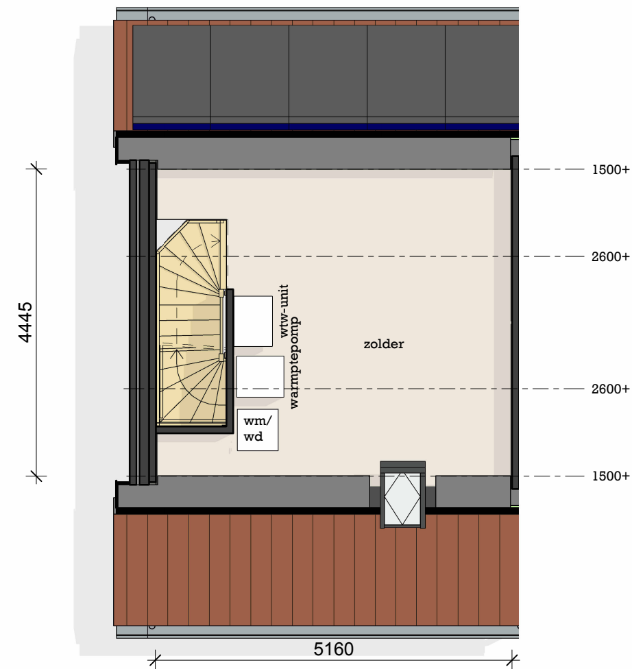
tweede verdieping
