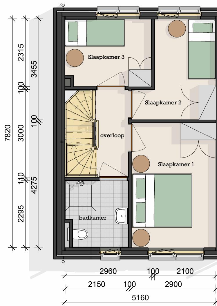
eerste verdieping
