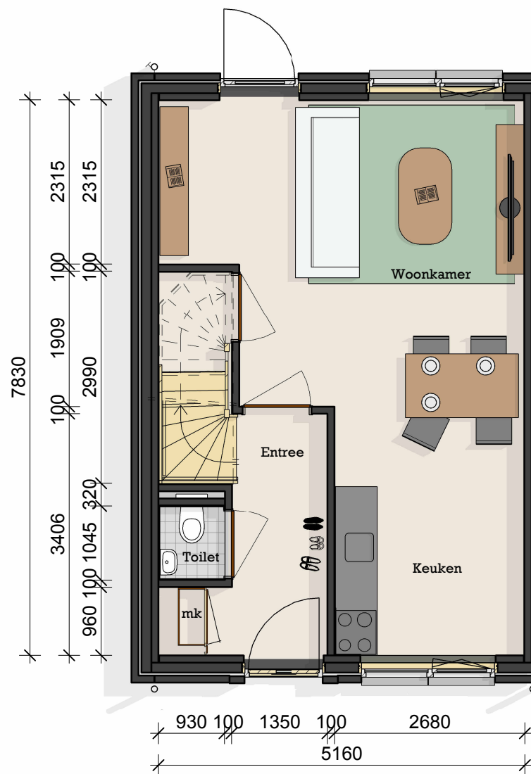
begane grond
